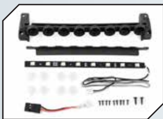
Art.Nr.: RC4VVVC1241 LED Lichtleiste für Dachträger für TRX-4 2021 Bronco (Rund)
